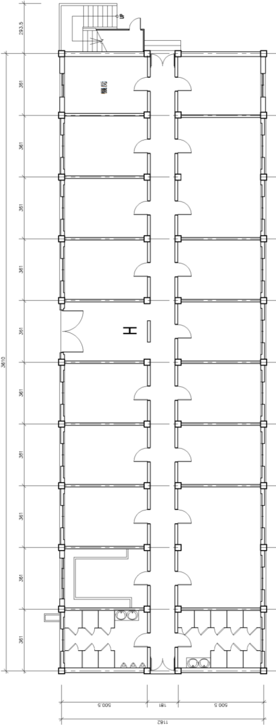
一層平面圖 S=1/150
